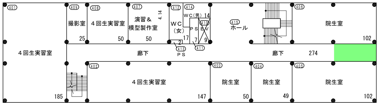
東1号館 4階平面図
