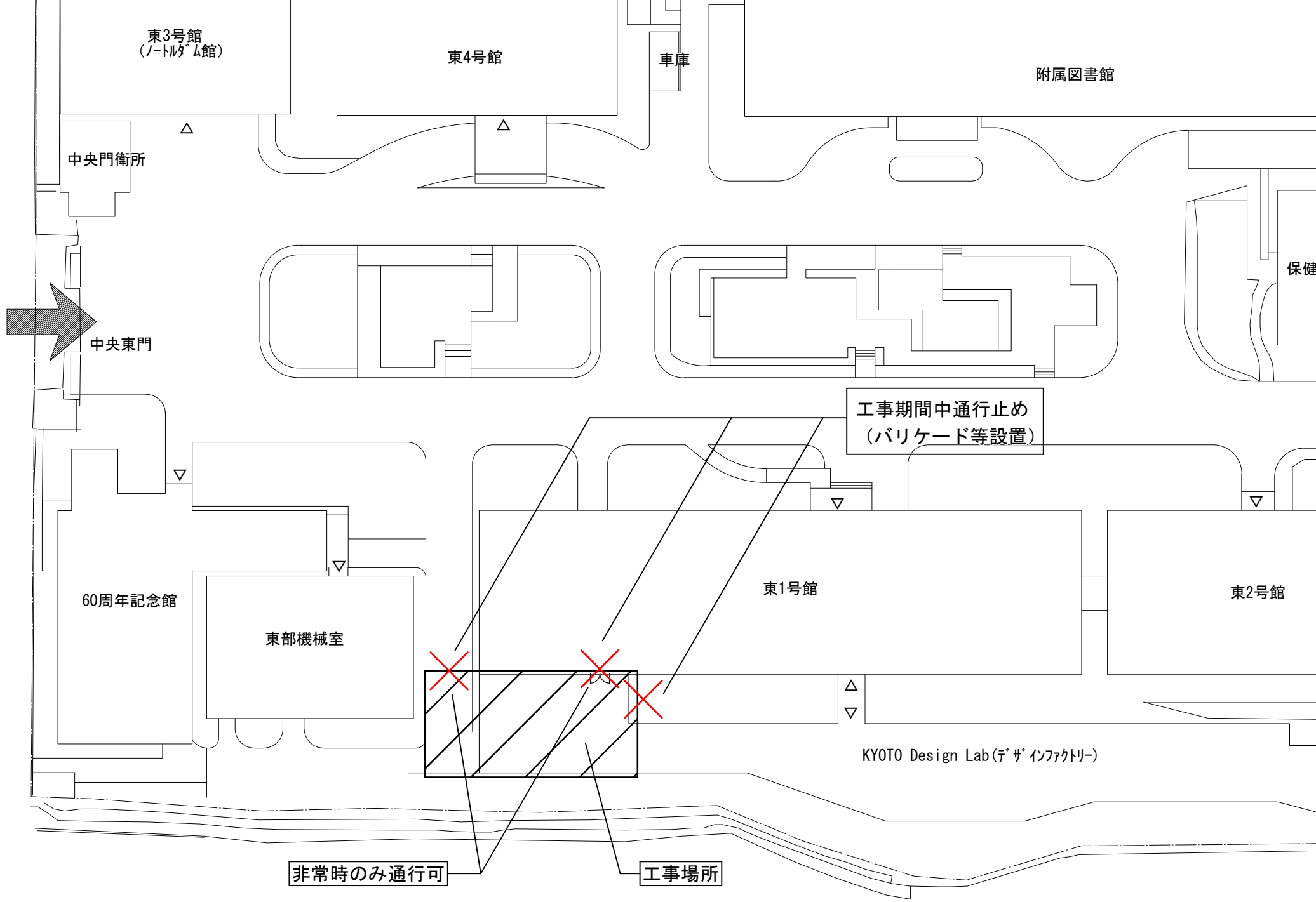
東構内 KYOTO Design Lab付近配置図
