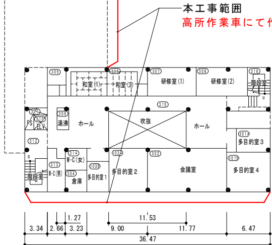
大学会館 3階平面図 1/400
