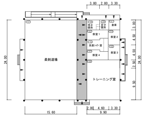
武道場・トレーニング室 1階平面図 1/400
