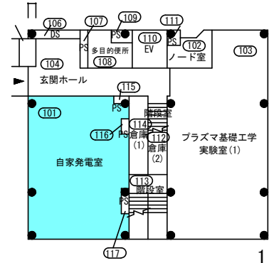
9号館 1階平面図
