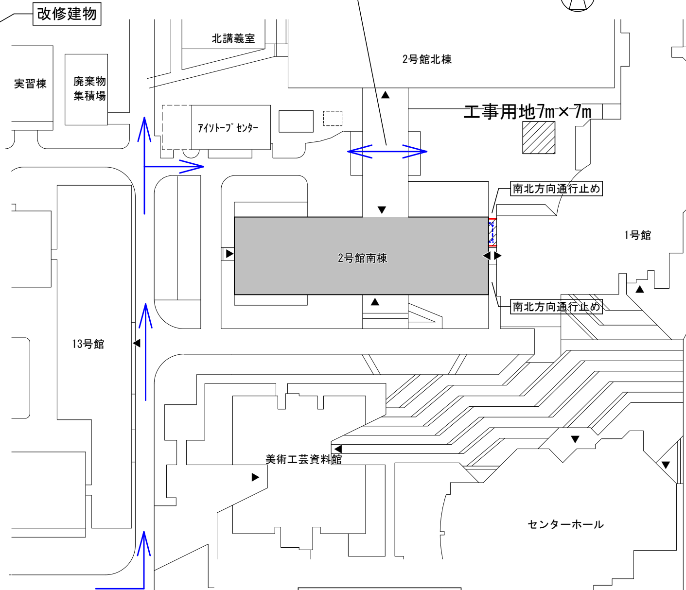
2号館南棟付近配置図 1/800
