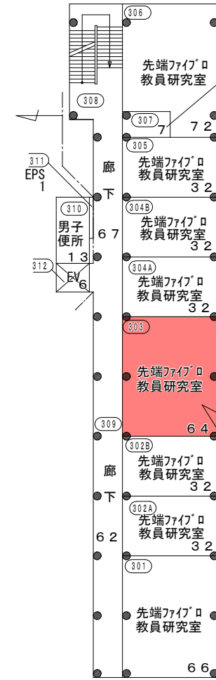
4号館3階平面図
