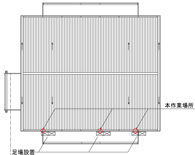
体育館 屋根伏図
