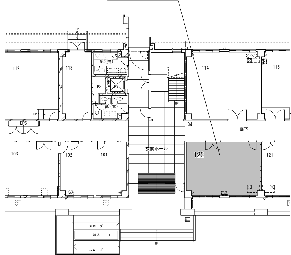
10号館 1階平面図 1/250
