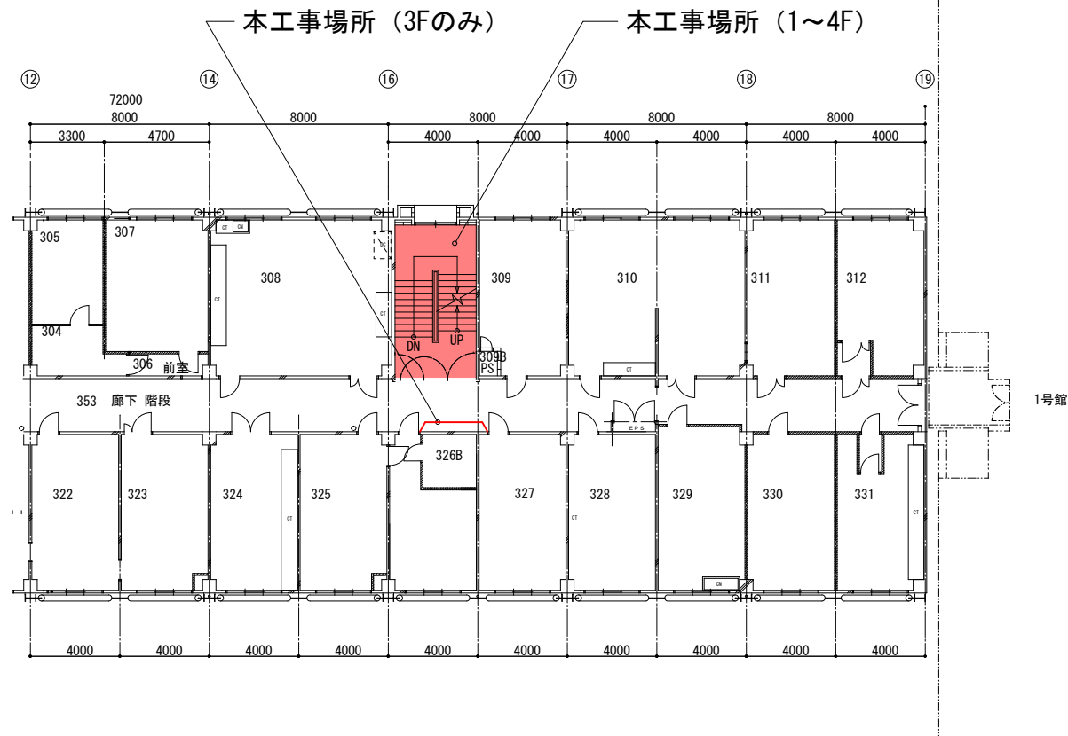
2号館北棟3階平面図 1/300
