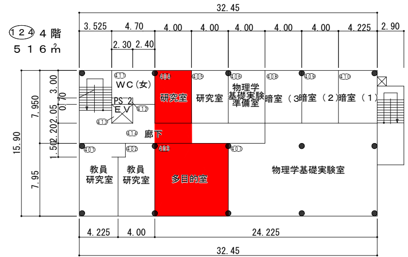
6号館4階平面図
