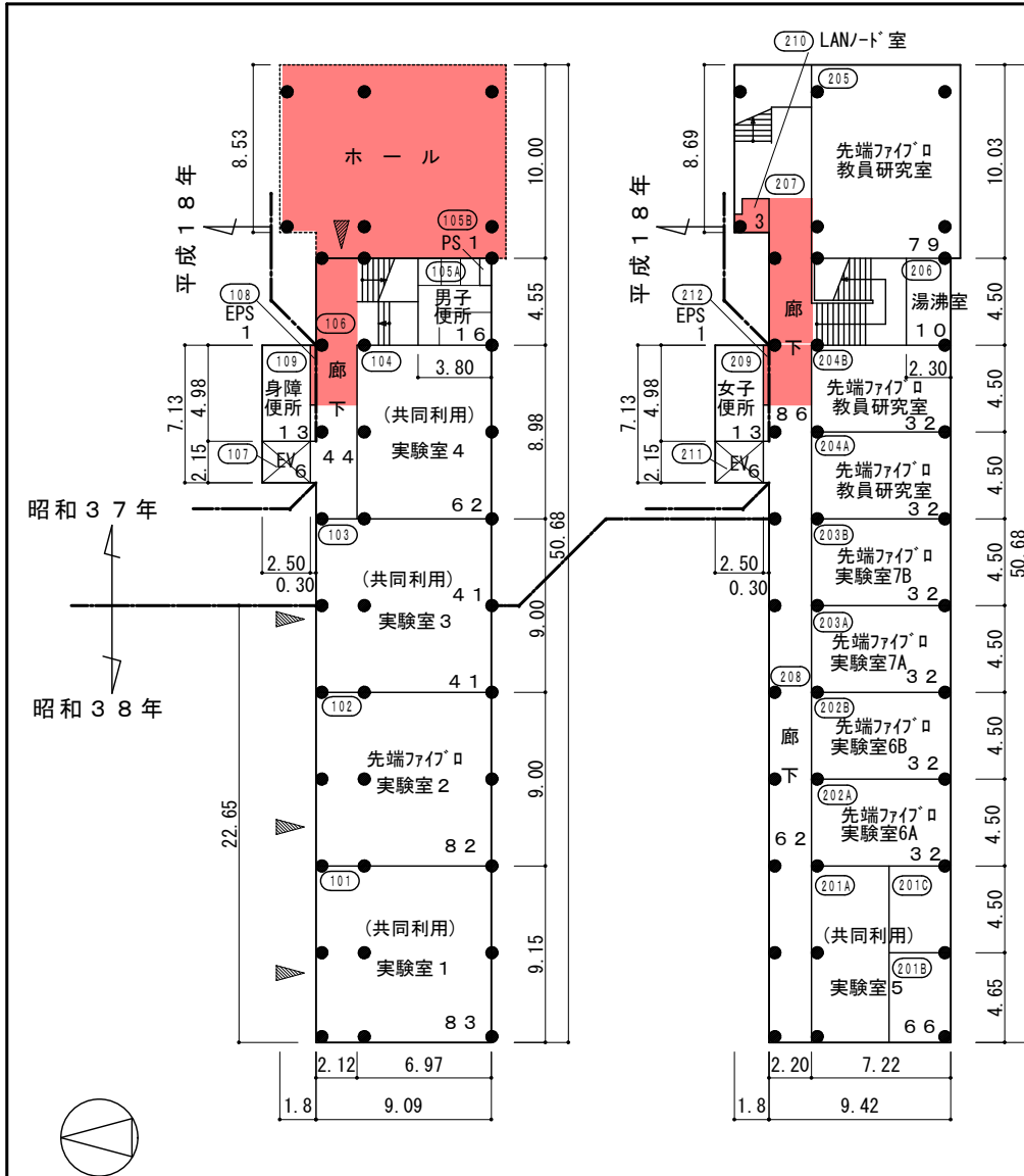
4号館1、2階平面図
