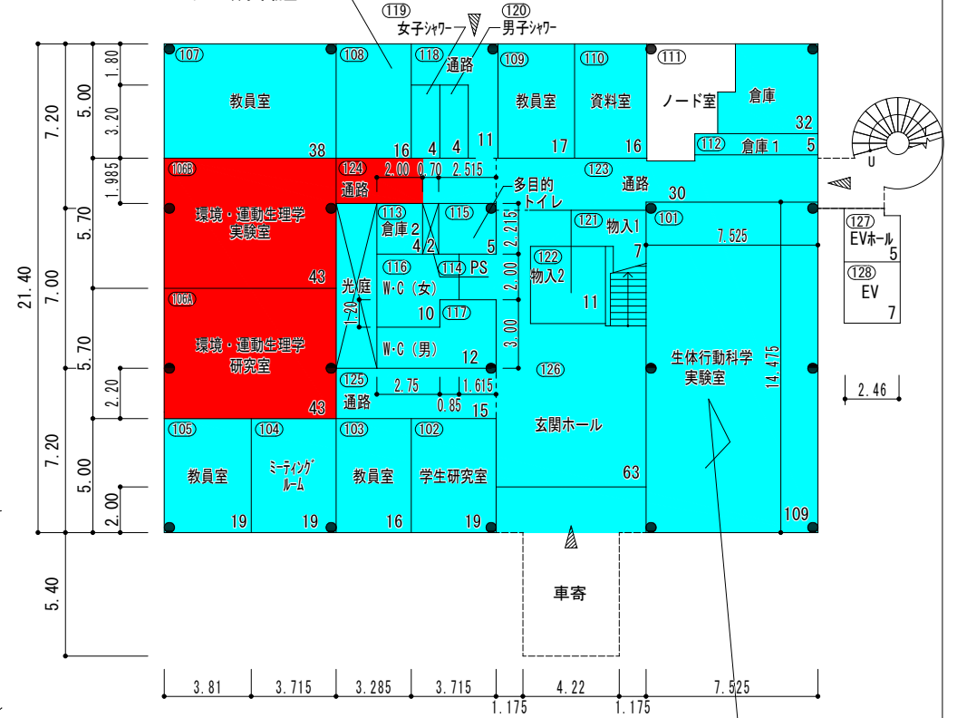
東4号館1階平面図
