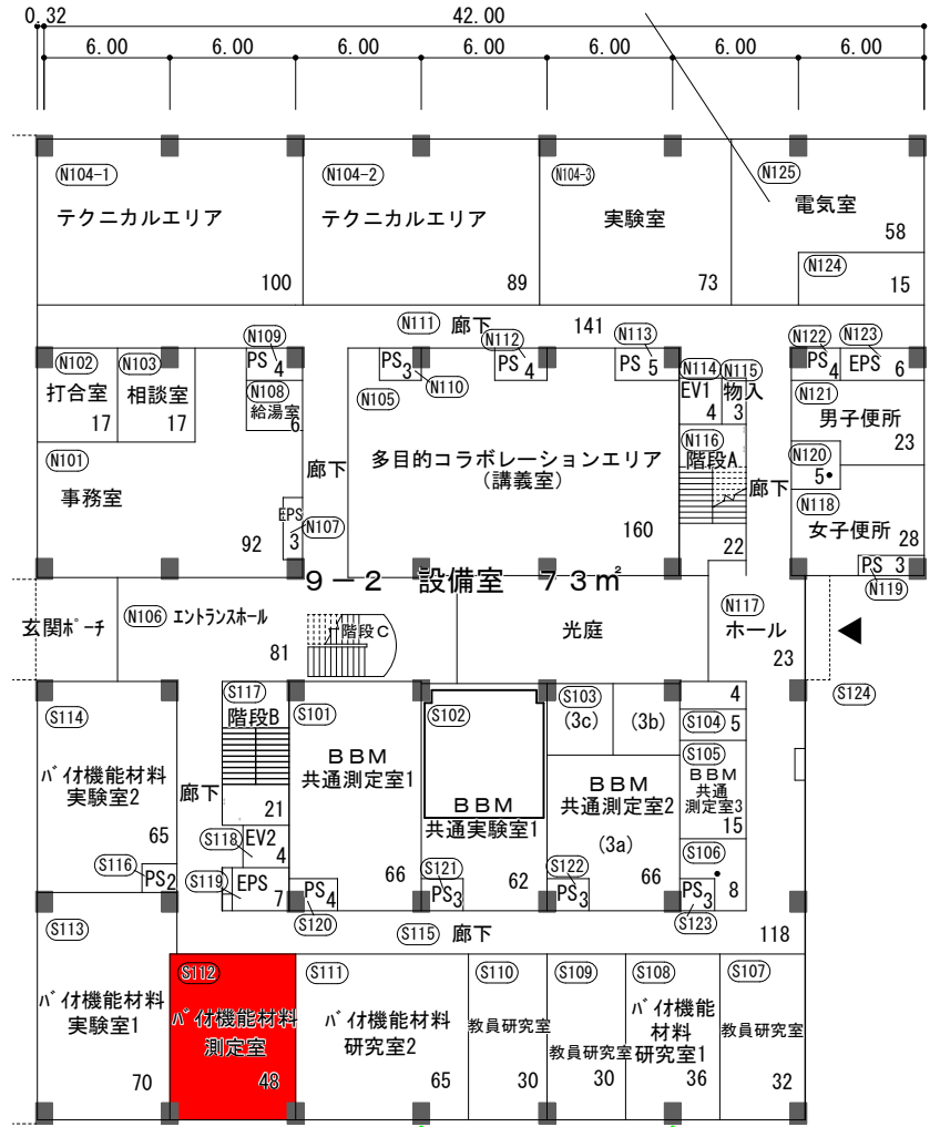
14・15号館1階平面図
