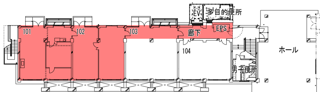
4号館 1階平面図
