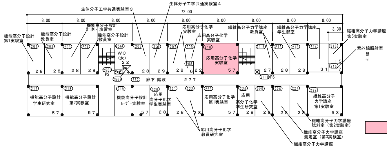
2号館北棟 2階平面図
