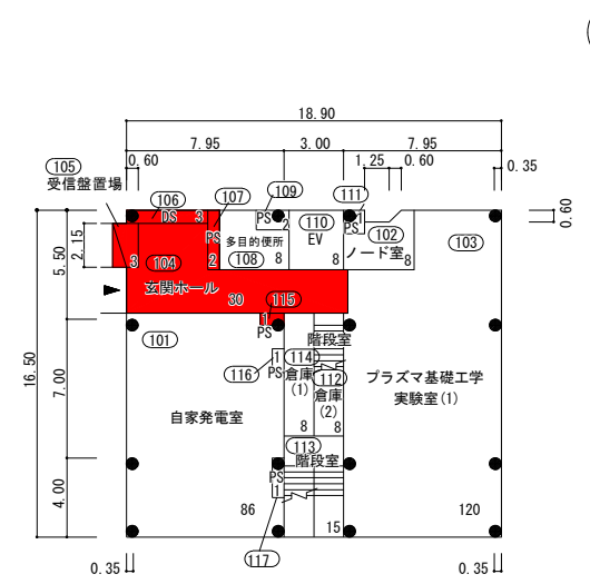
9号館1階平面図 (1/300)
