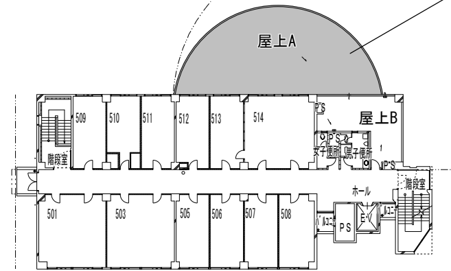
1号館 5階平面図
