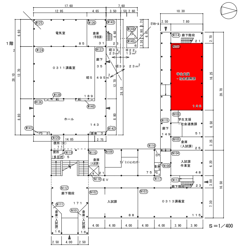
3号館1階平面図(北側)
