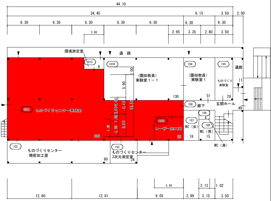
西実験棟 1階平面図
