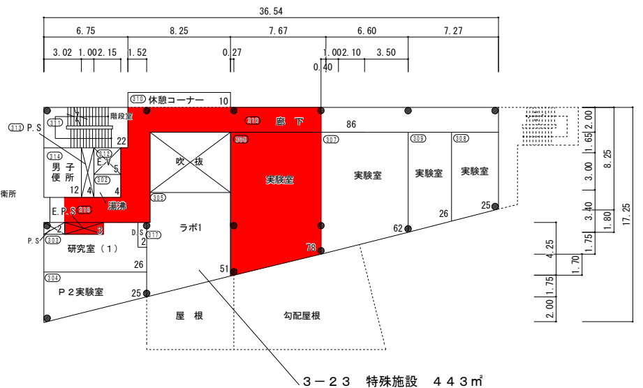
16号館3階平面図 (1/300)
