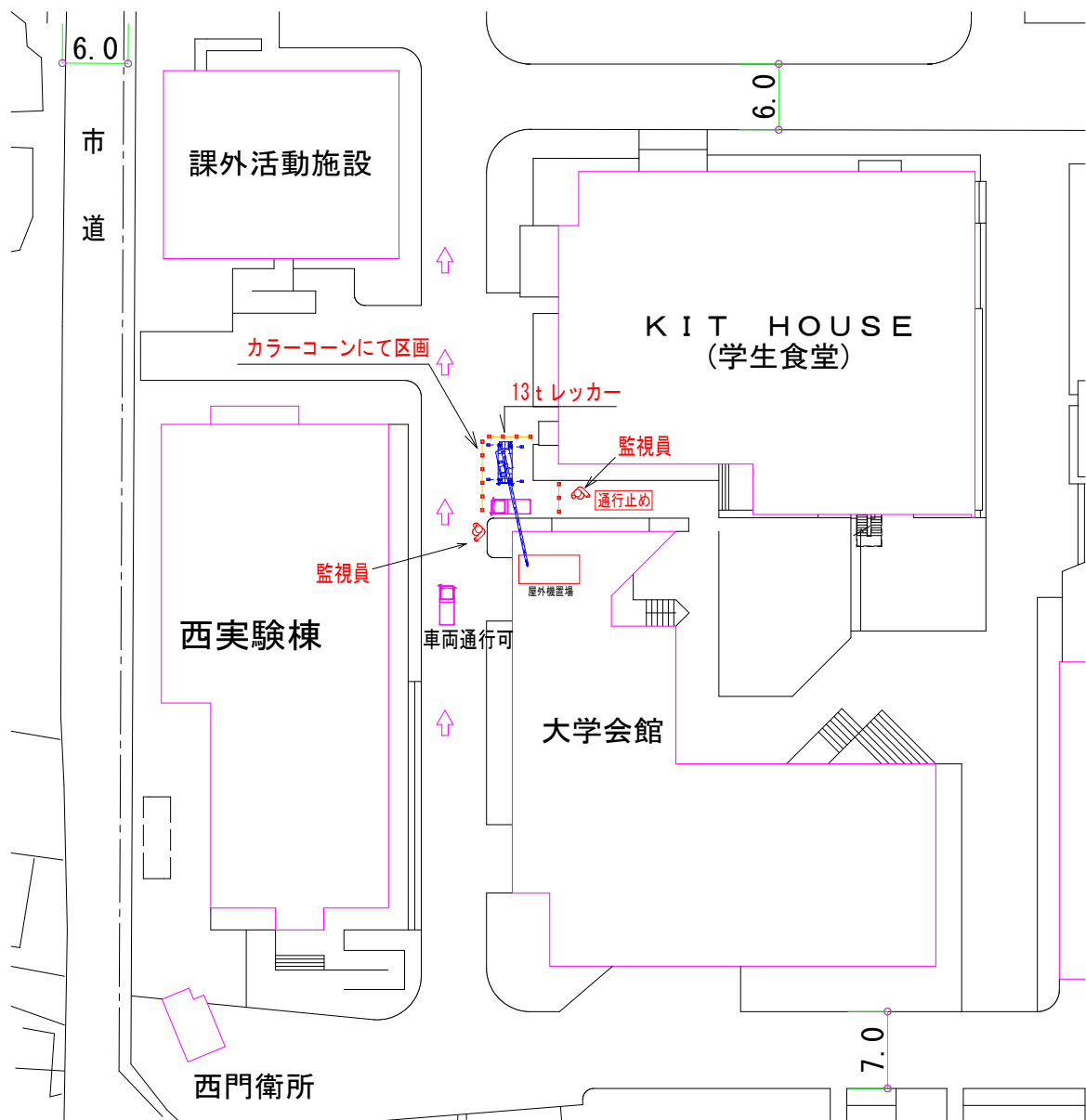
レッカー作業計画図
