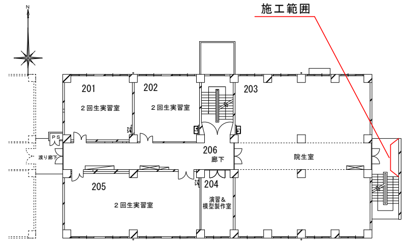
東2号館 2階平面図
