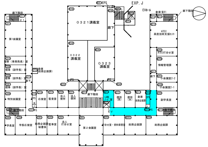
3号館2階平面図
