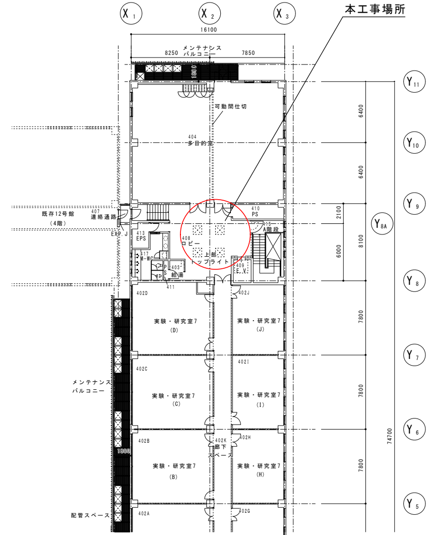
13号館4階平面図 1/400
