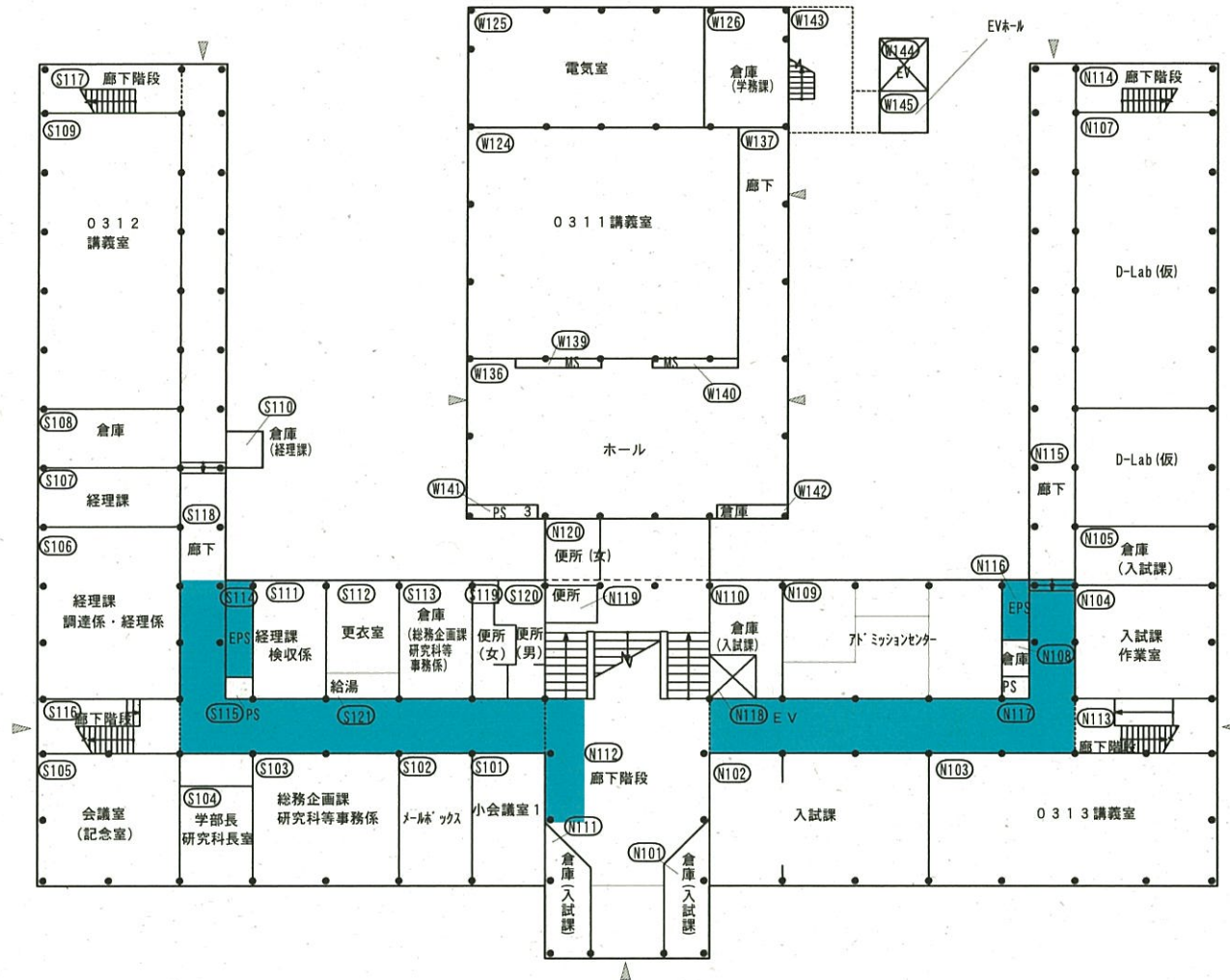
3号館1階平面図
