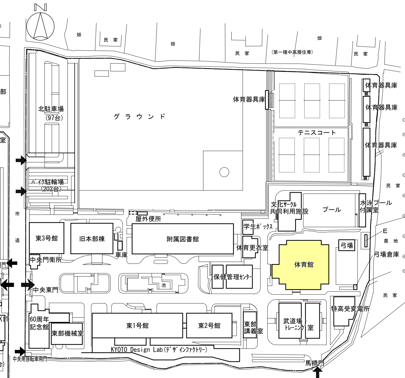
松ヶ崎団地東構内図
