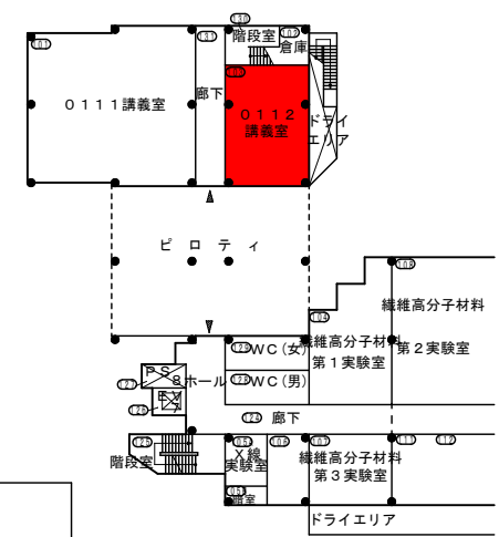
1階平面図
