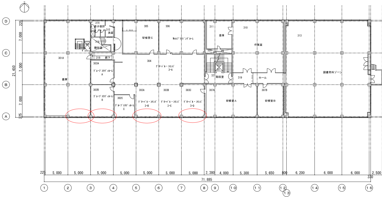
附属図書館3階平面図 1:200
