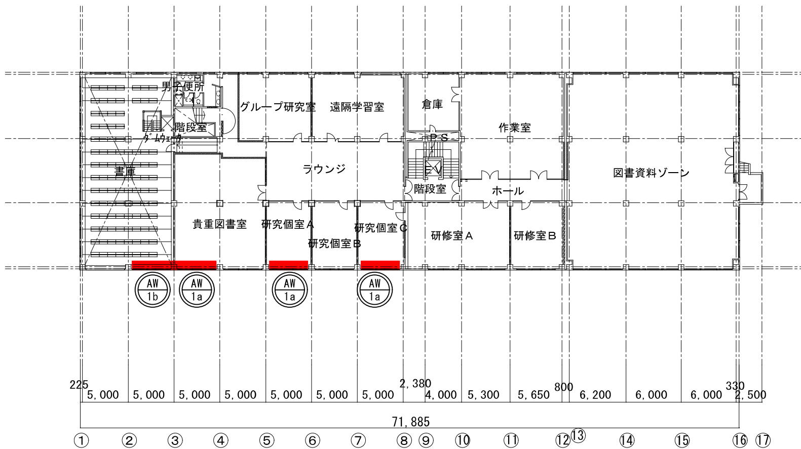
図書館 3階平面図
